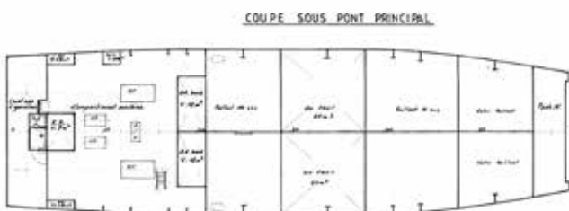
COUPE SOUS PONT PRINCIPAL
