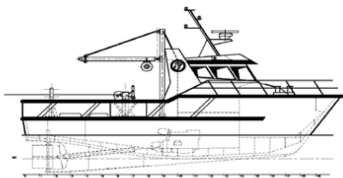
VUE LONGITUDINALE
